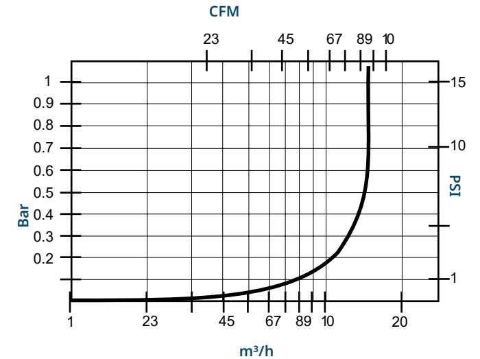
■ Air Discharge
