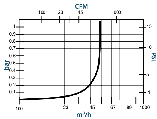
■ Air Discharge
